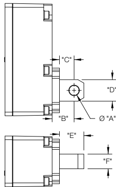
Rear Eye (KSRE-60, KSME-60)
